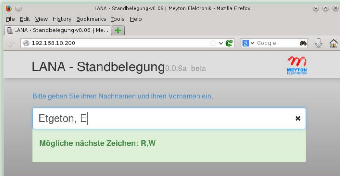
Abbildung 7: Vorschlag der nächsten möglichen Zeichen
